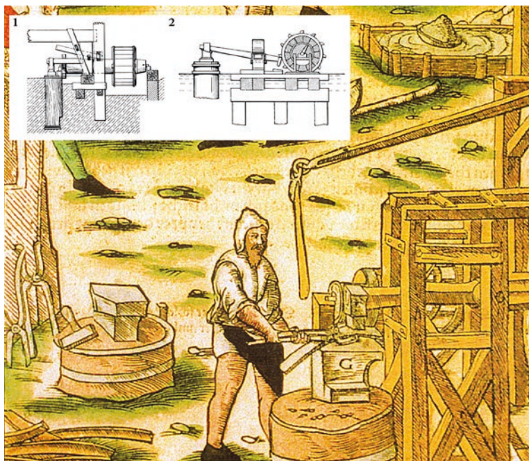
Ryc. 2 – młot: 1 – podrzutowy, 2 – naciskowy (wg Georgius'a Agricola)
