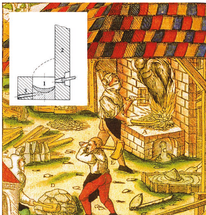
Ryc. 1 - dymarka niska: 1 - zaprawa, 2 - ścianka ogniowa, 3 - lacher (wg Georgius'a Agricola)
