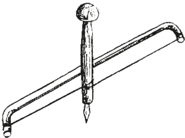
Przyrząd do wiercenia otworów w toporkach (za G. Childe)
